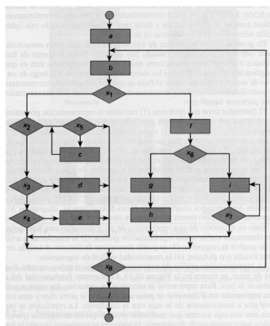
Figura 10. Un diagrama de flujo estructurado
