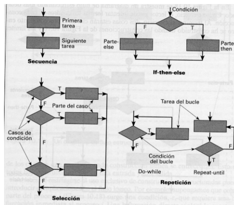
Figura 9. Construcciones de programación estructurada con diagramas de flujo
