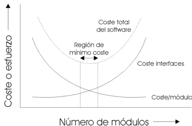
Figura 3. Modularidad y coste del software
