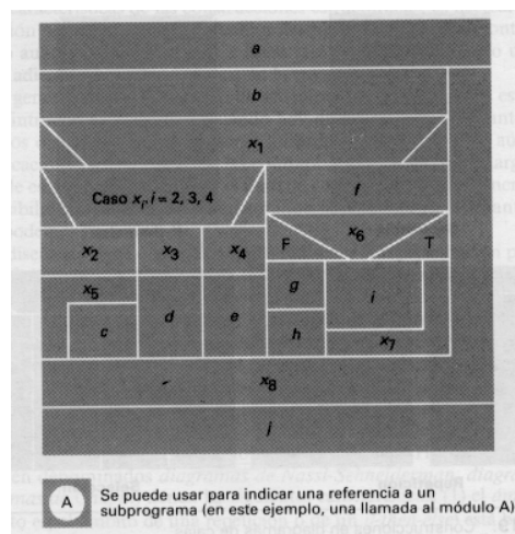
Figura 12. Un diagrama de cajas estructurado
