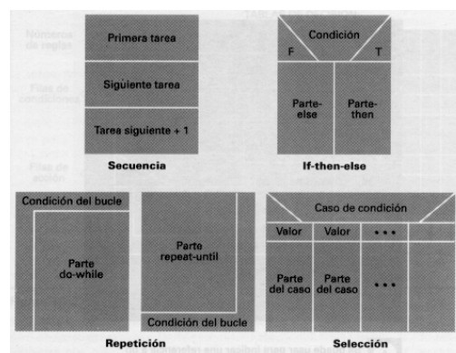
Figura 11. Construcciones en diagramas de cajas
