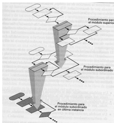
Figura 7. Procedimiento realizado por capas
