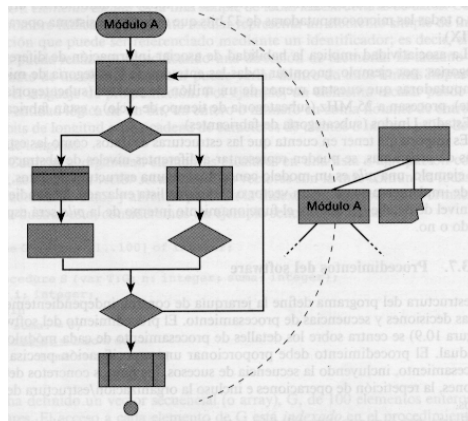
Figura 6. Procedimiento dentro de un módulo
